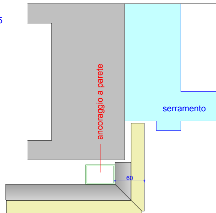
PARTICOLARE CHIUSURA SU SERRAMENTO
