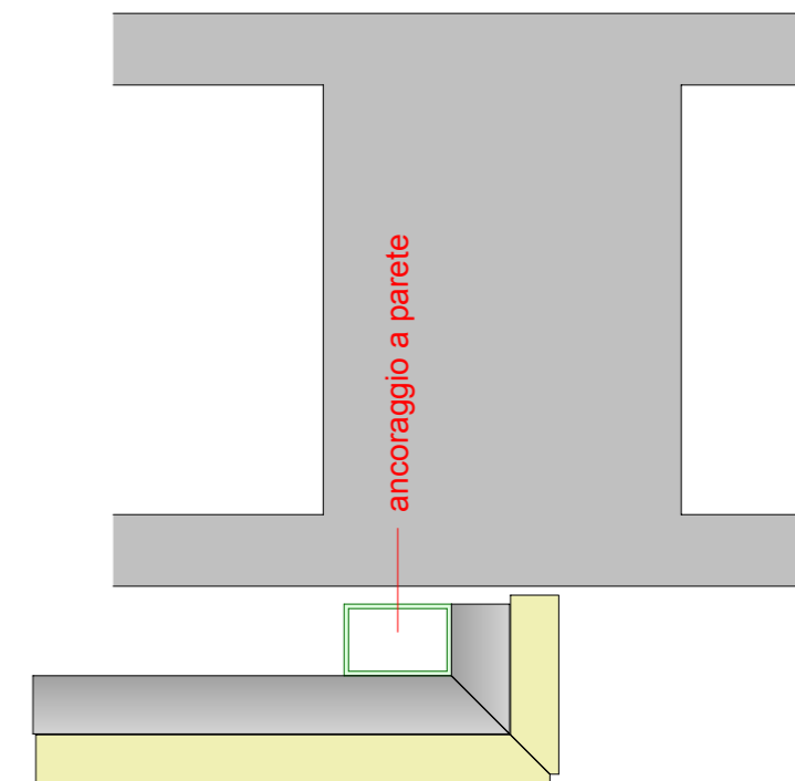
PARTICOLARE CHIUSURA SU MURATURA
