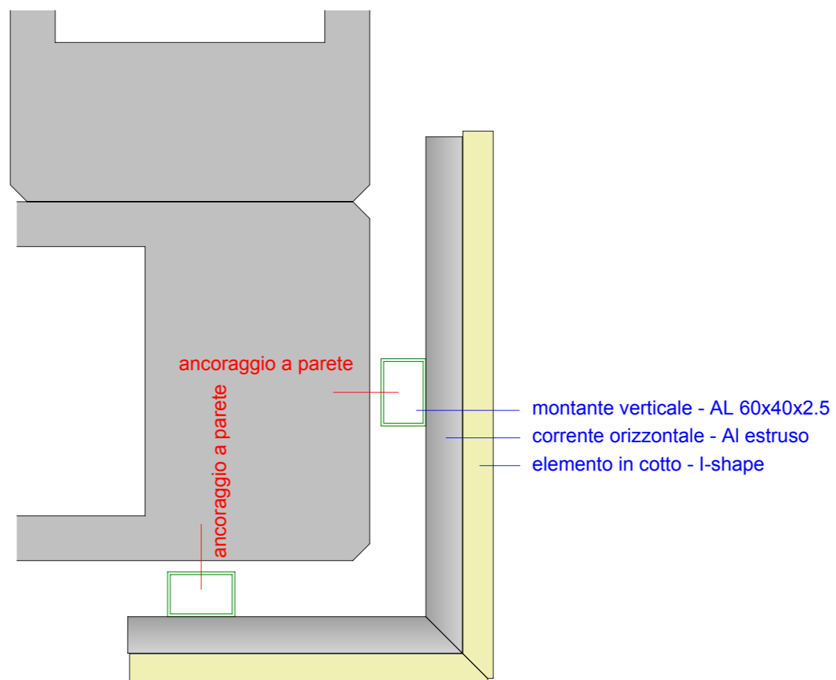
PARTICOLARE ANGOLO
