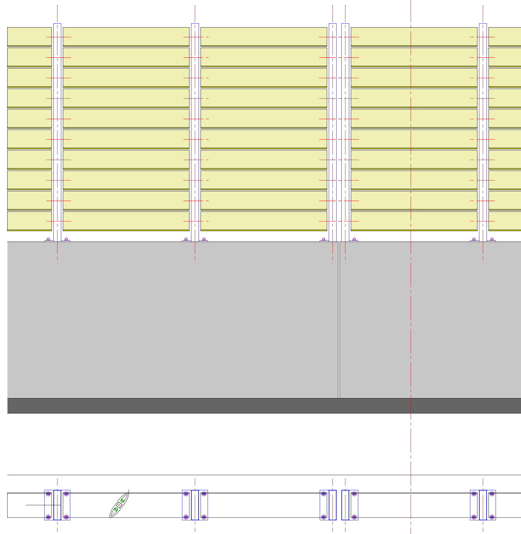
modulo tipo giunto
