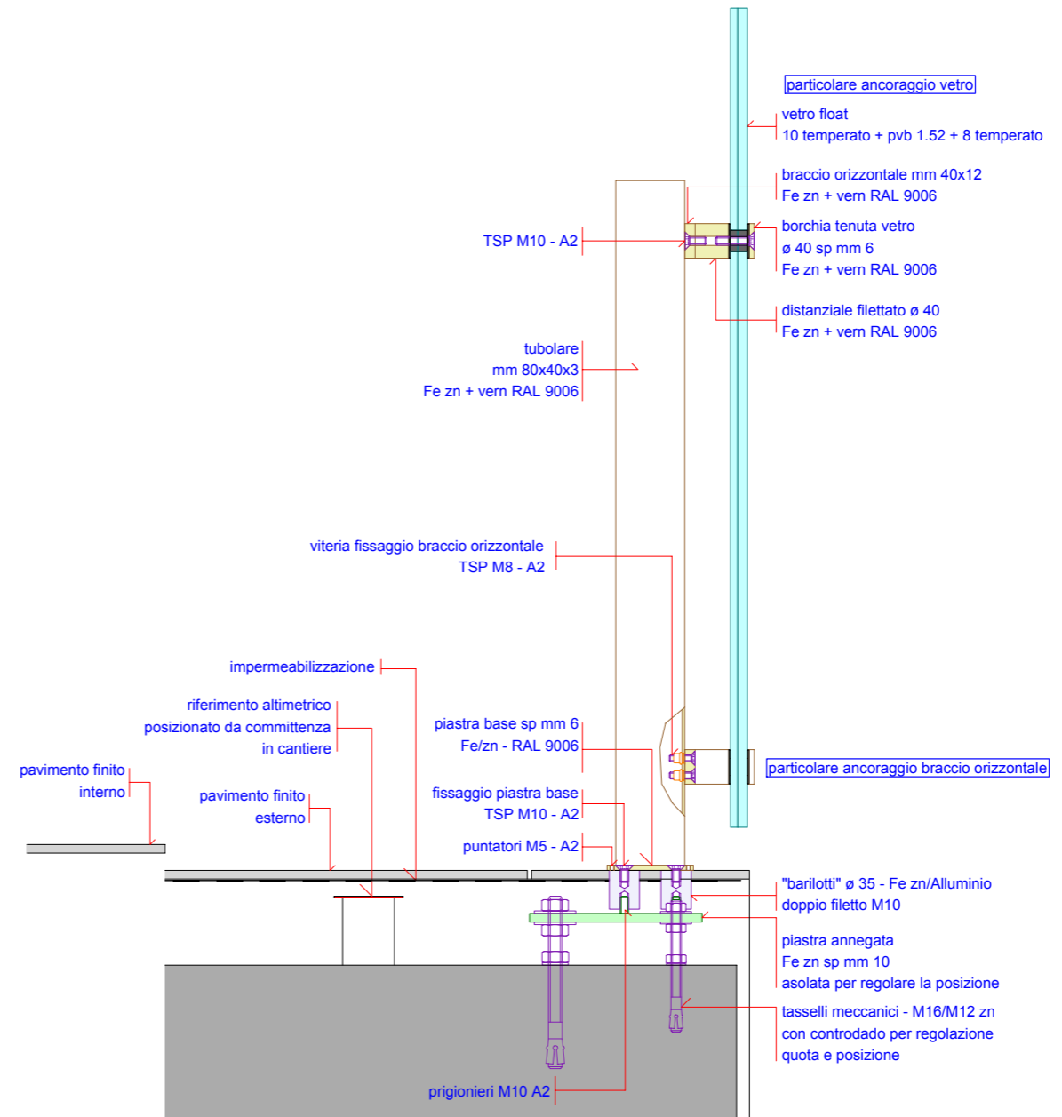
sezione
